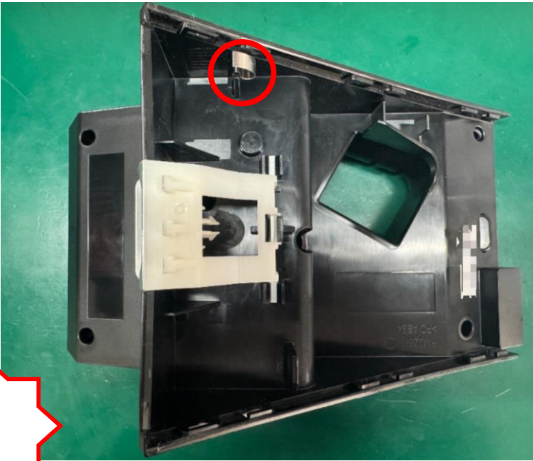
图一，检查 MC359 没有变形或者损坏。
