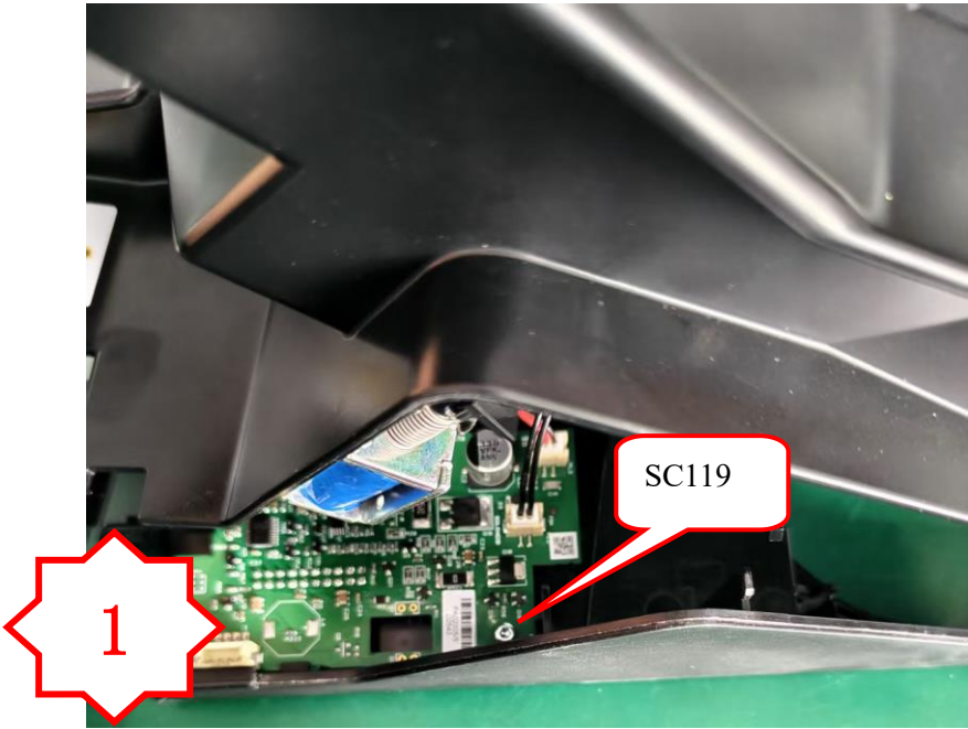
图一，用电批将 SC119 螺丝拆出
