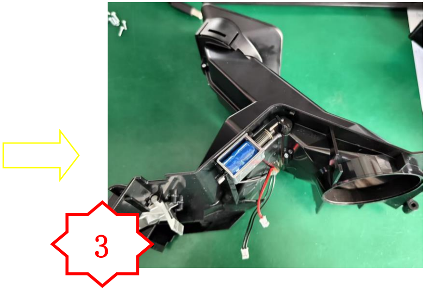
PA1153 组件的螺旋管贴上透明胶固定后待出货
