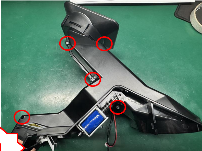
图一，检查五颗螺丝是否打到位。
