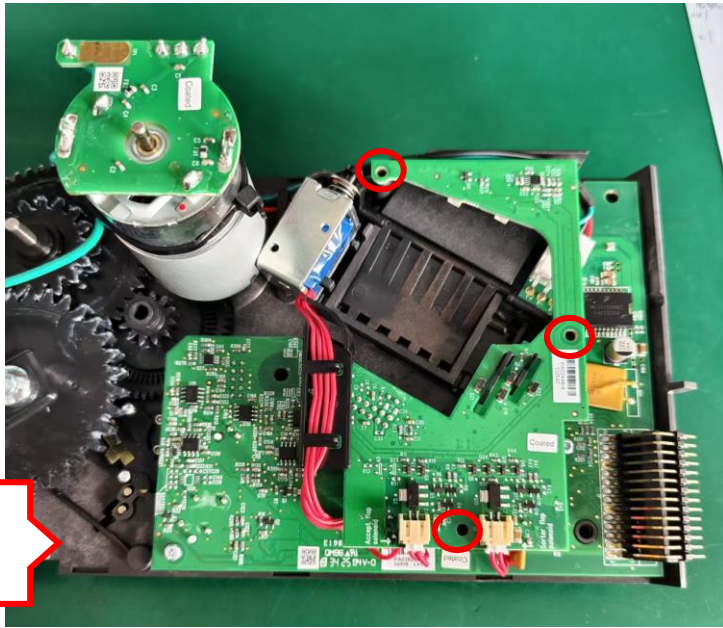
图一， 用电批取出 3 个 SC119
