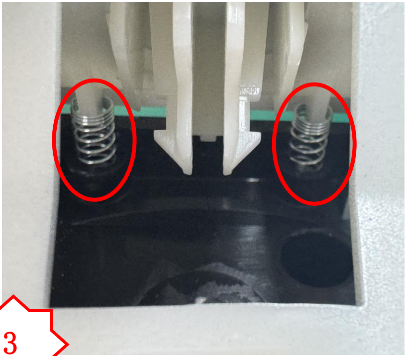
图一，检查 MC359 没有变形或者损坏。
